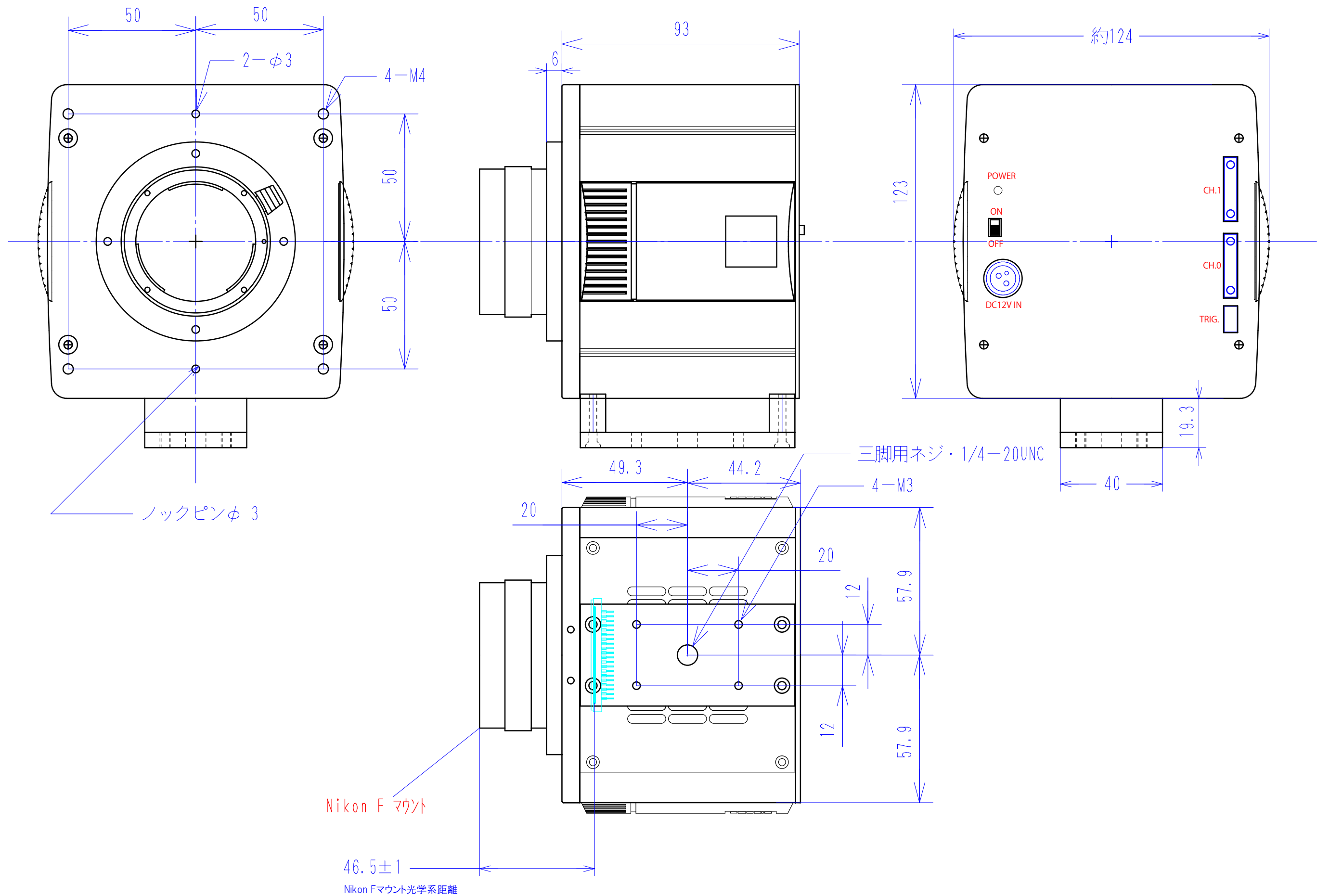
BH-60M/BH-65M 外觀寸法図
